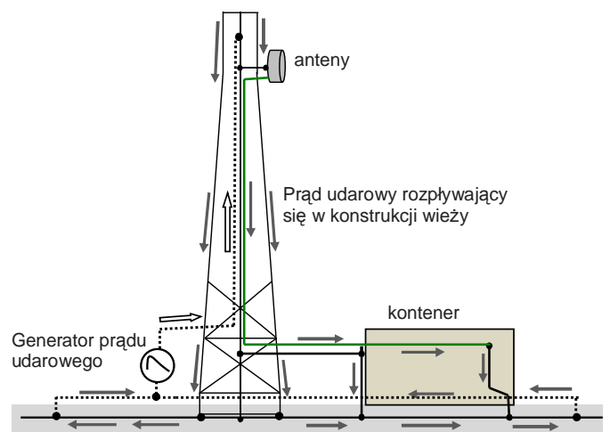
Rys. 6. Układ połączeń do badania zagrożeń piorunowych stacji bazowej [5]
