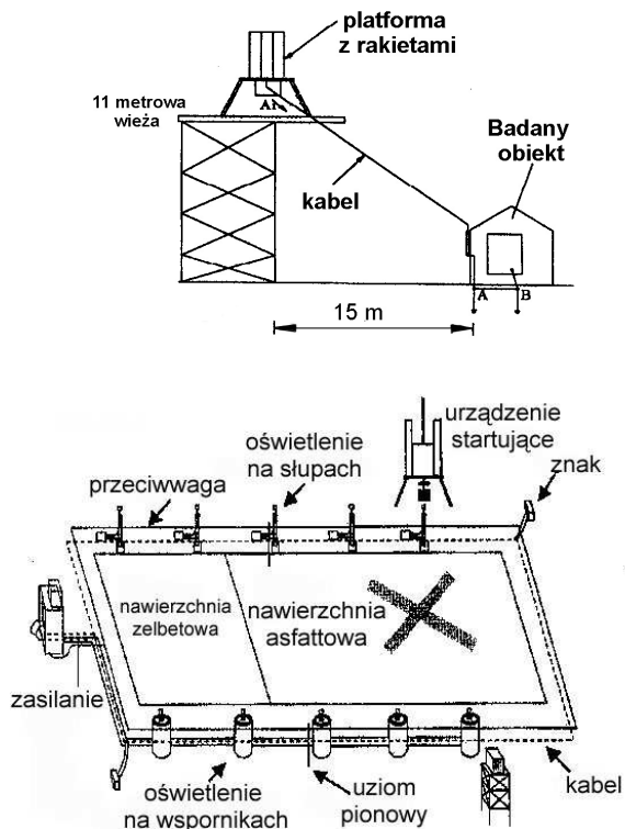
Rys.2. Układy do badań zagrożeń wywołanych przez prowokowane wyładowania piorunowe
