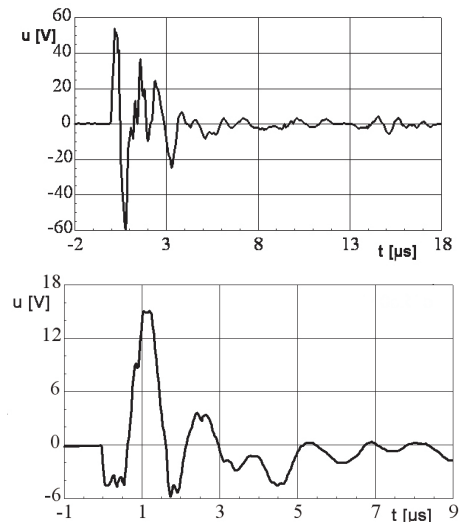
Rys. 5. Przykładowe przebiegi napięć indukowanych w gniazdach sieci komputerowej
