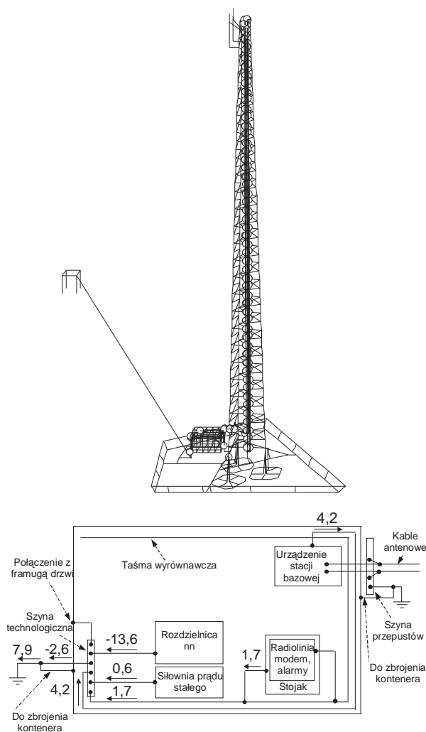
Rys. 10. Model matematyczny stacji bazowej oraz przykład wyznaczonego rozplywu prądu udarowego w kontenerze podczas wyładowania w wieżę
